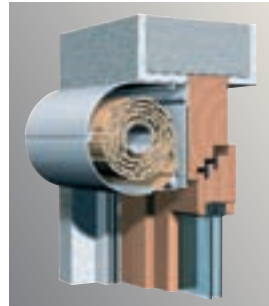
Rund-Rollladen Rund-Optik als gezielter Blickfang
