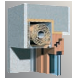
Putzträger-Variante Ob Rollladen oder Raffstore – hinter dem Putz nahezu unsichtbar, und trotzdem perfekte Dämmung durch die Positionierung außen
